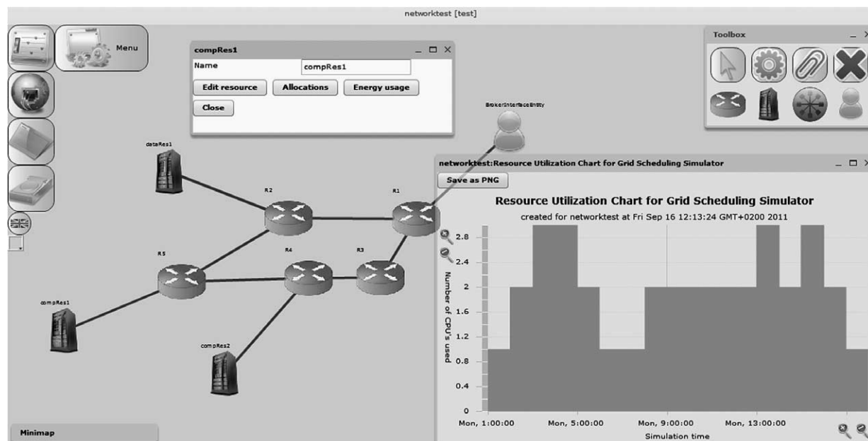
Fig. 6. GSSIM GUI.
